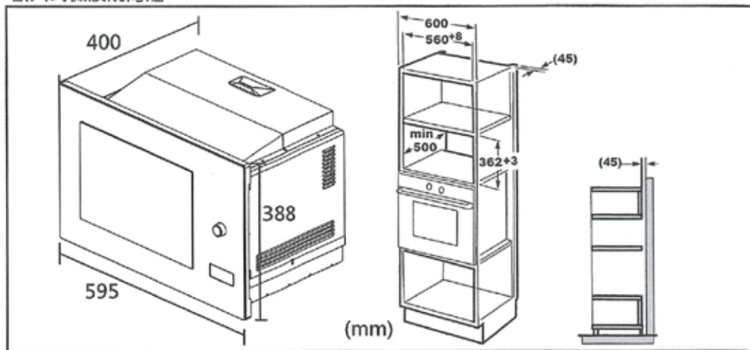
AK-BMW925 嵌入式微波燒烤爐
